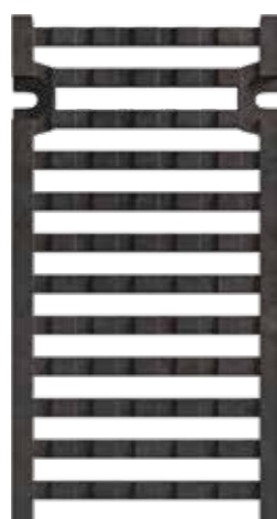
GRIGLIA IN GHISA SFEROIDALE ANTITACCO D.M 236/89 C 250 E D 400 dimensioni: 20x200x500 mm
