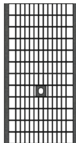
GRIGLIA ZINCATA ANTITACCO D.M 236/89 MAGLIA 30x10 B 125 dimensioni: 20x200x1000 mm
